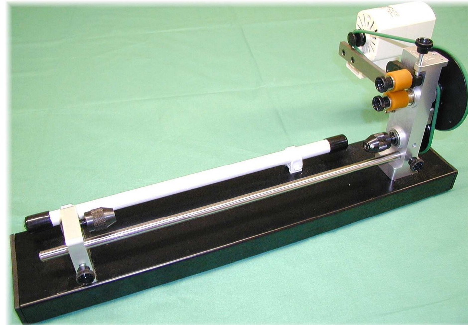
Die Maschine mit stufenlosem elektrischem Antrieb, läuft mittels Fußpedal extrem langsam an. Sie haben beide Hände frei zum Arbeiten.
