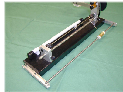
Wickelführung 38.- €
